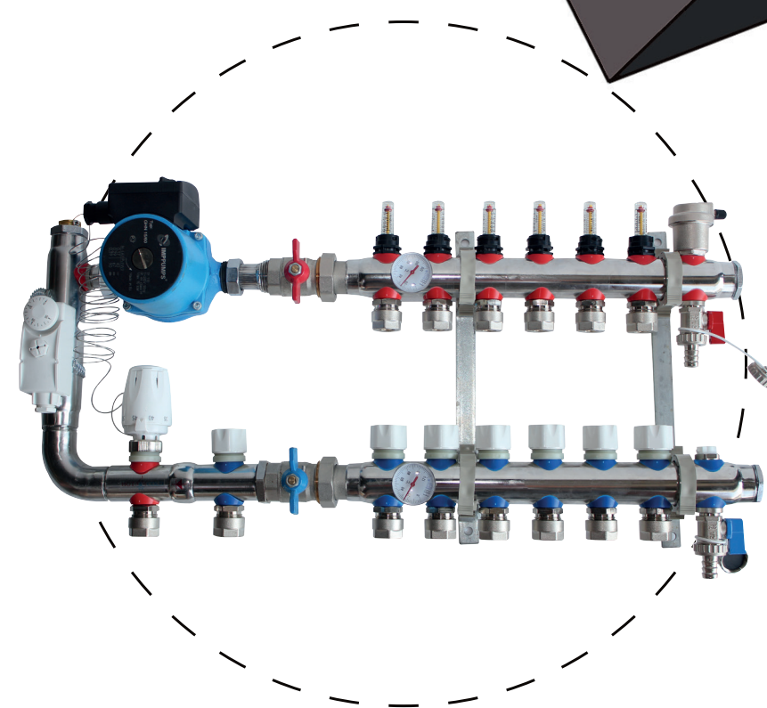
RVS complete verdeler/verzamelaar "comfort"
